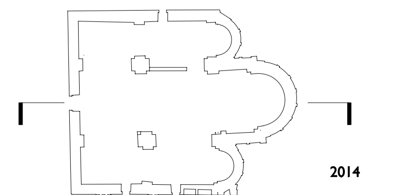
ESGLÉSIA DE SANT PERE DE CASSERRES SECCIÓ LONGITUDINAL A SUD
