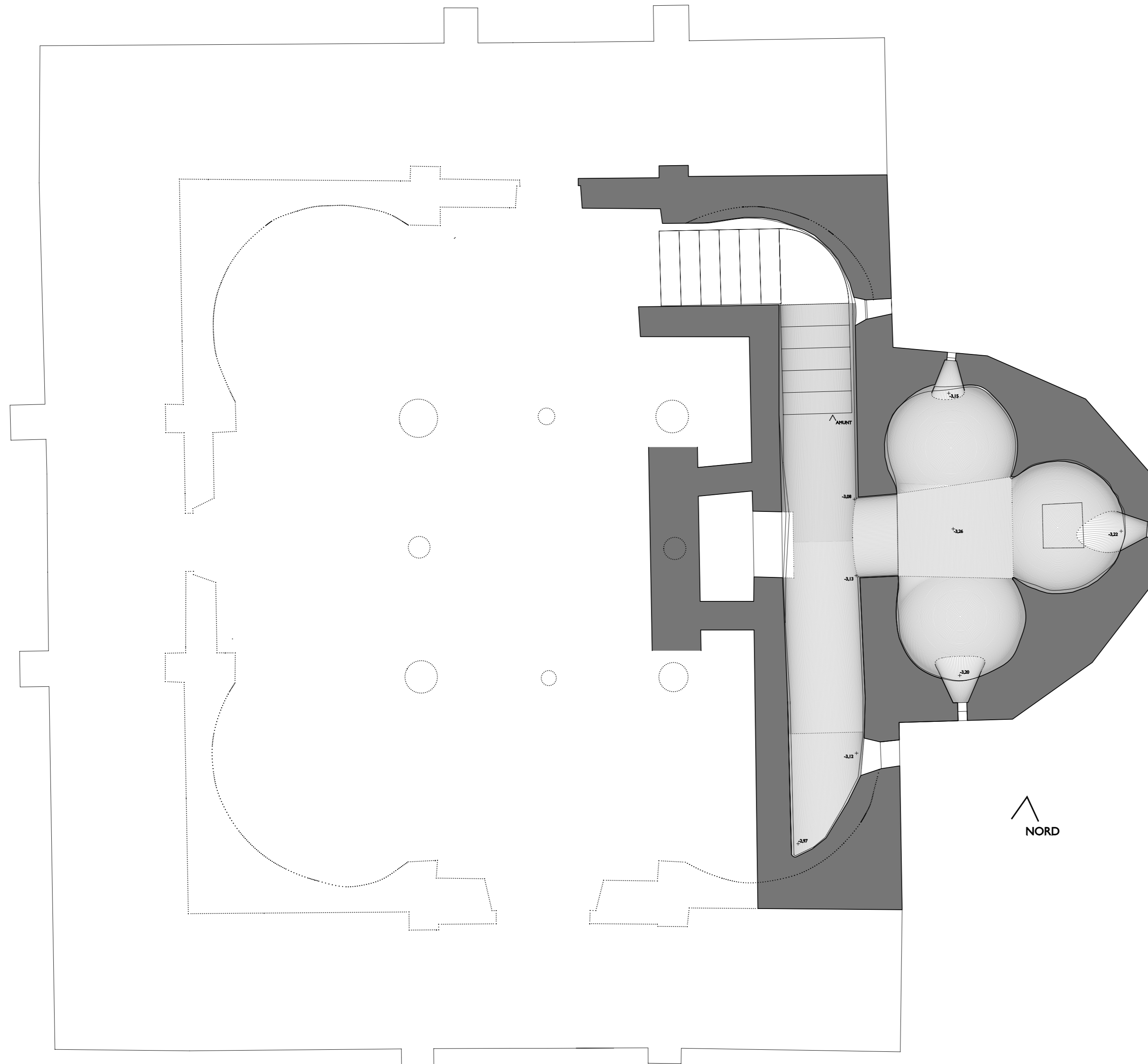
ESGLÉSIA DE SANT MIQUEL, SANT PERE DE TERRASSA PLANTA A NIVELL DE LES FINESTRES DE LA CRIPTA
